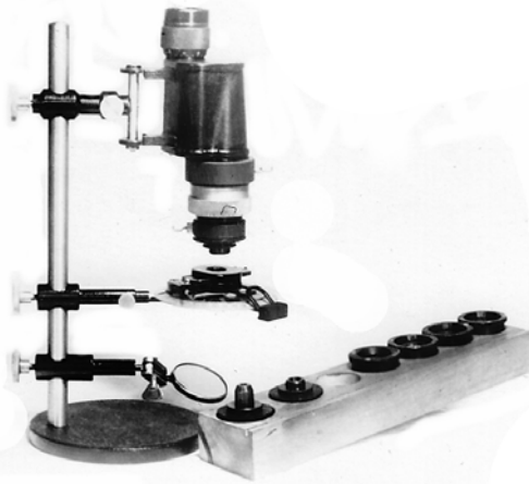
Микроскоп и лупа для работы геолога в поле
