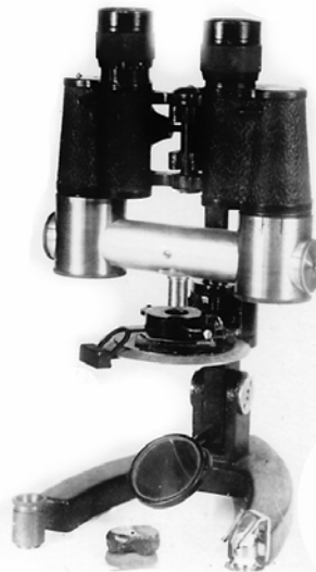
Биноклярный однообъективный минералогический микроскоп
